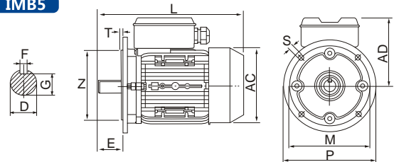
IMB5
